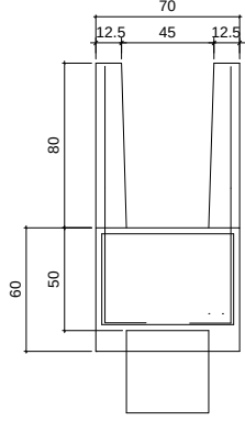
Corte BB
