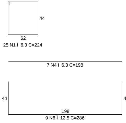
Corte AA
