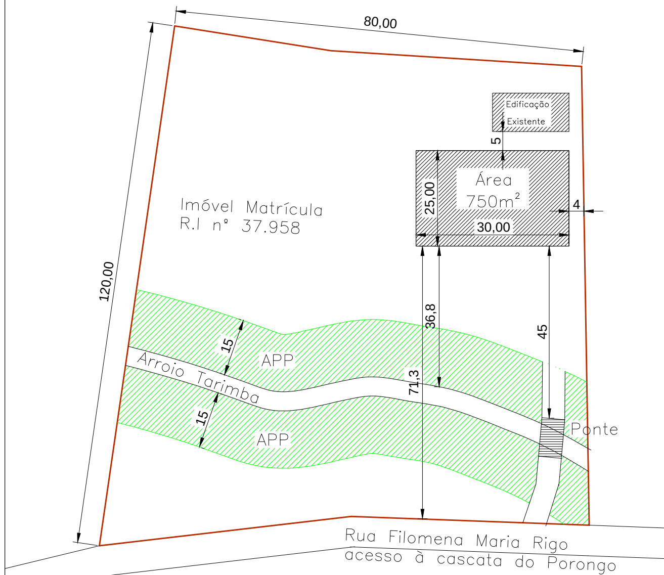
01 PLANTA DE LOCALIZAÇÃO ESC.: s/e
