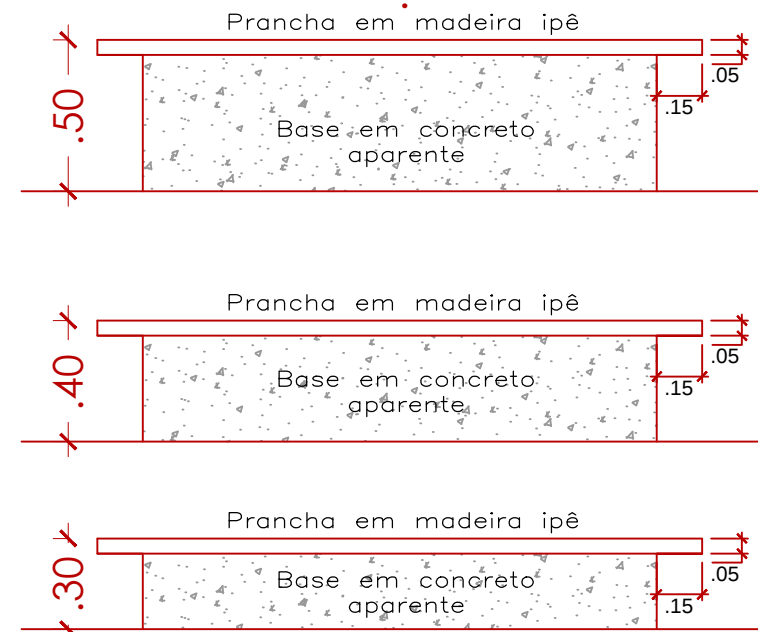
Detalhe 2- Bancos 1/25
