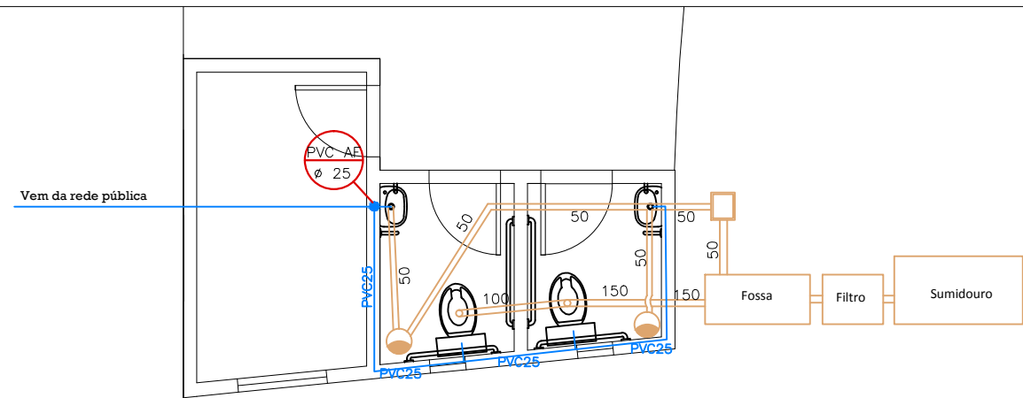
1 Hidrossanitário - Apoio Esc. 1/75
