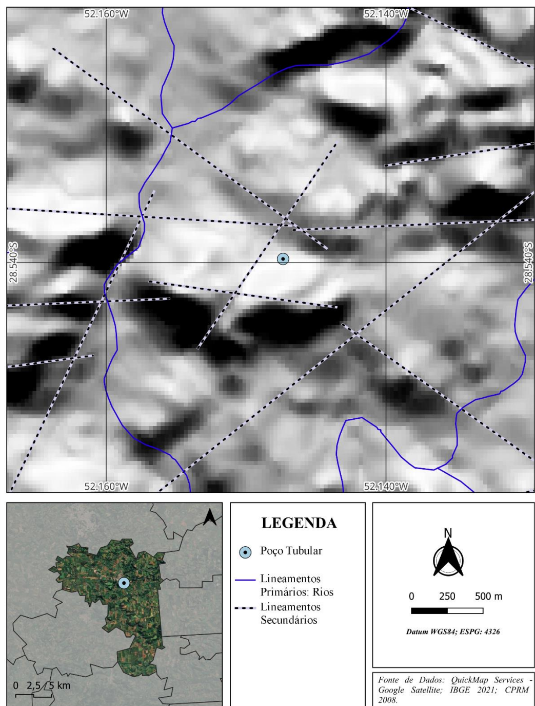
Figura 2: Lineamentos primários e secundários no possível ponto de locação do poço tubular.
