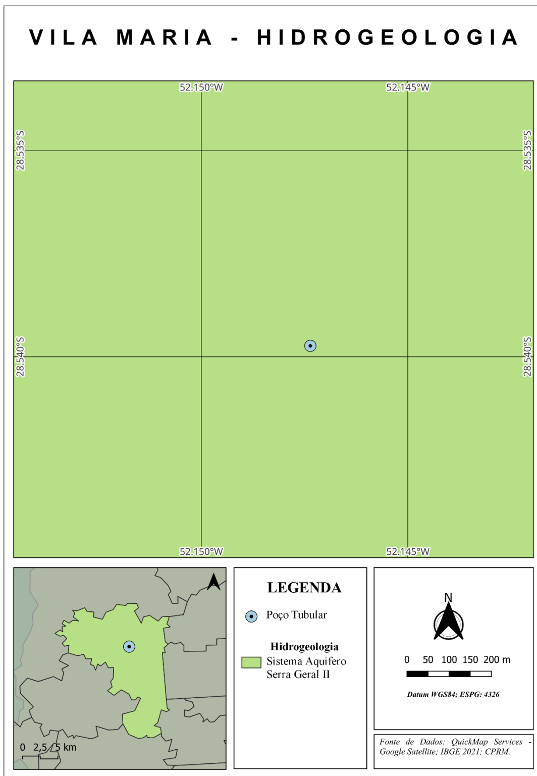
Figura 4: Tipo de aquífero encontrado na possível área de locação.
