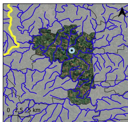
Figura 3: Hidrografia regional: ênfase para a Bacia dos Rios Taquari-Antas..
