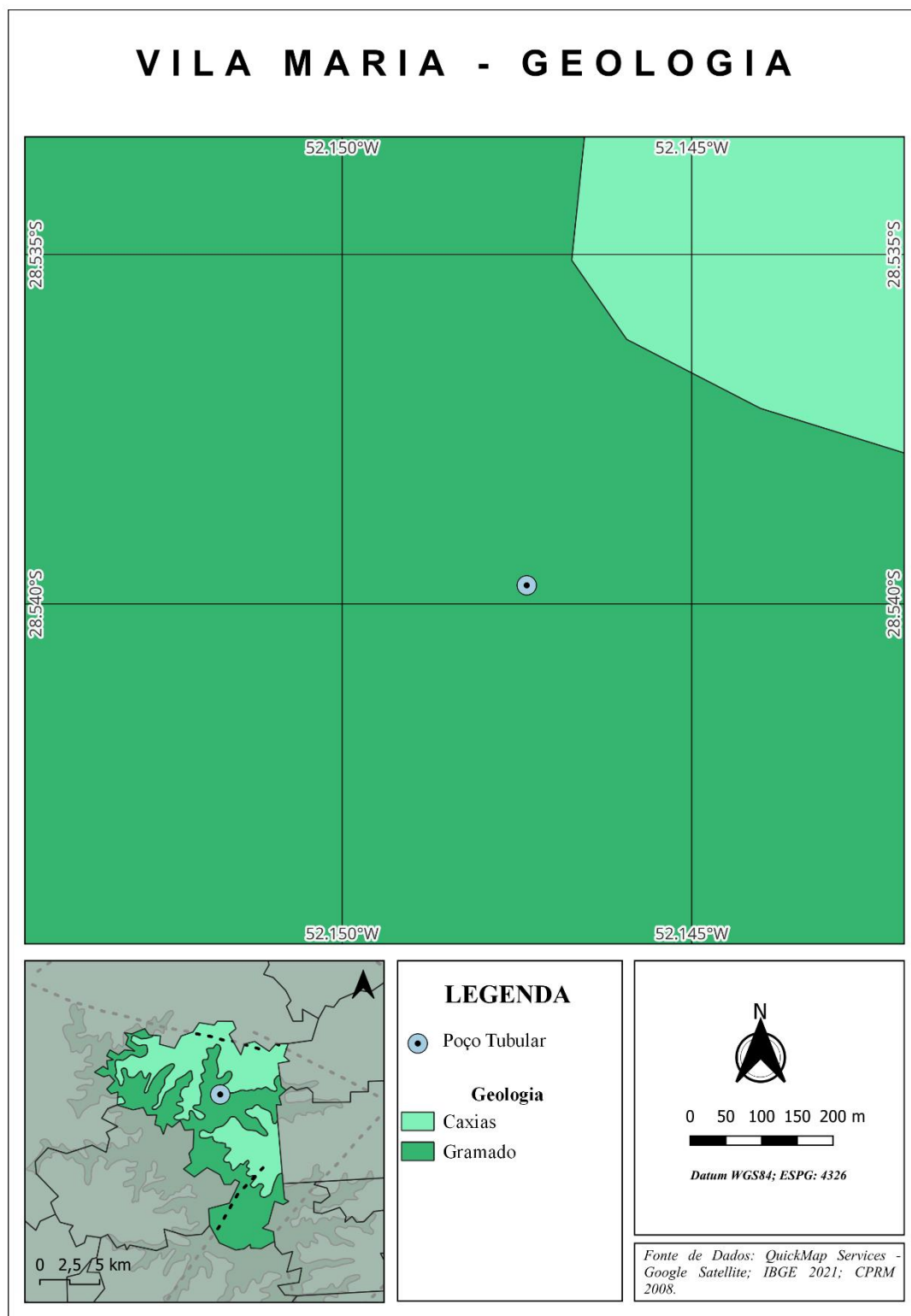
Figura 1: Mapa Geológico da área para locação de poço tubular na cidade de Vila Maria/RS,
