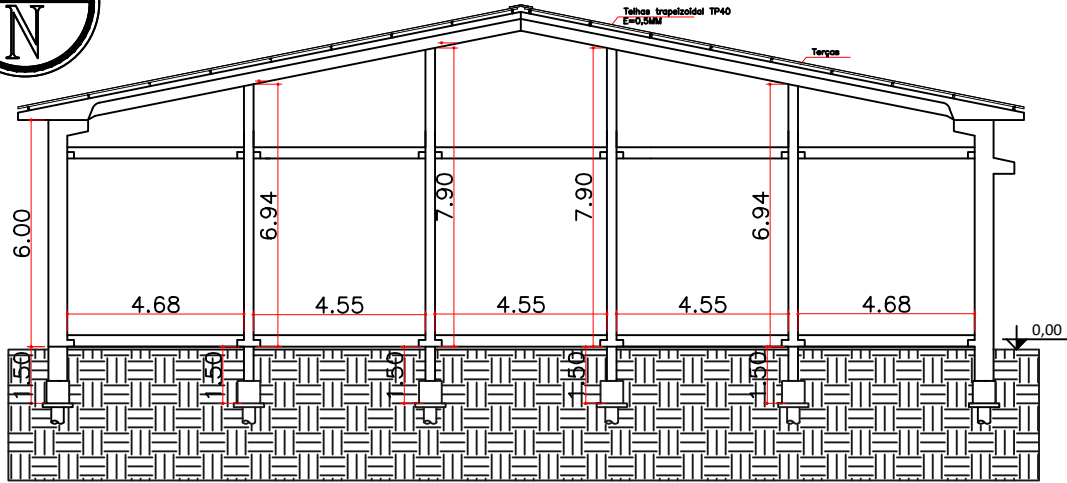
04 CORTE AA ESC.: 1/200
