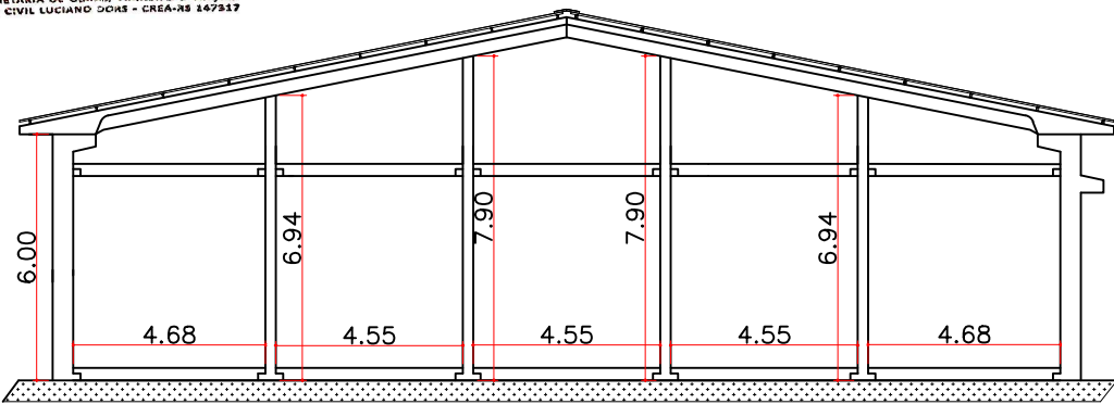
06 FACHADA ESC.: 1/200
