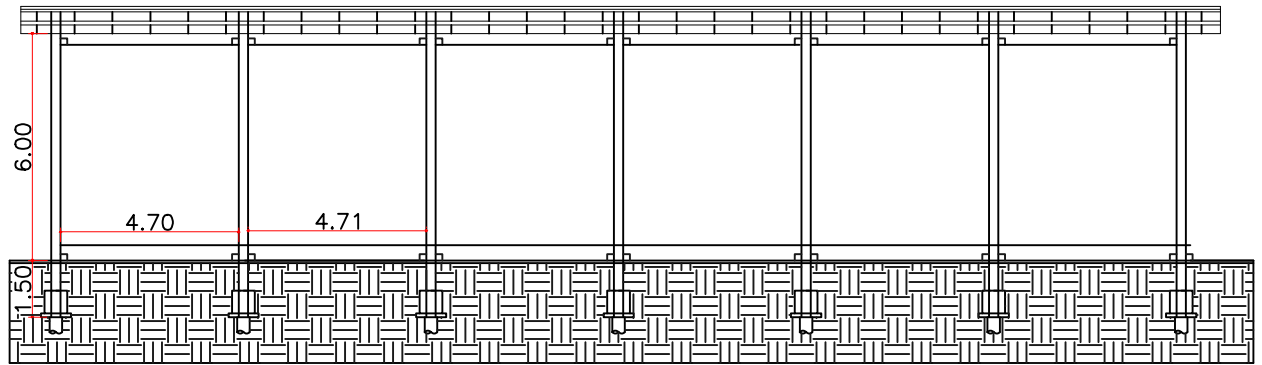
05 CORTE BB ESC.: 1/200
